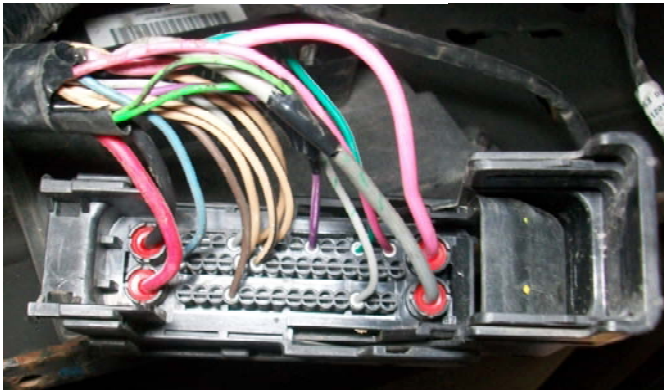
47 ПИНовый разъем БЛОКА УПРАВЛЕНИЯ БЕНЗИНОВОГО НАСОСА
