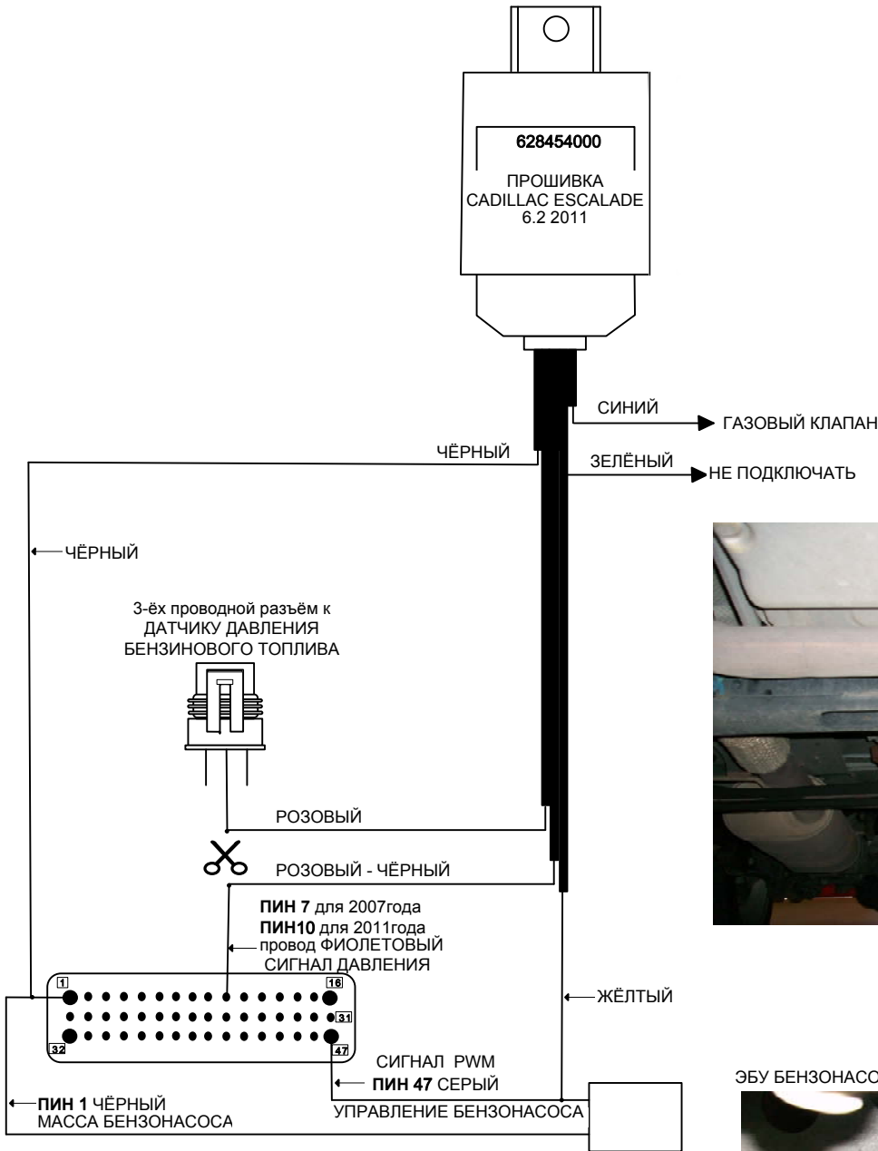
47 ПИНовый разъем БЛОКА УПРАВЛЕНИЯ БЕНЗИНОВОГО НАСОСА
